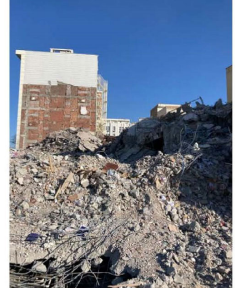
Enkaz alanı ve aynı adada bulunan ve yıkılmayan 7 katlı bina
