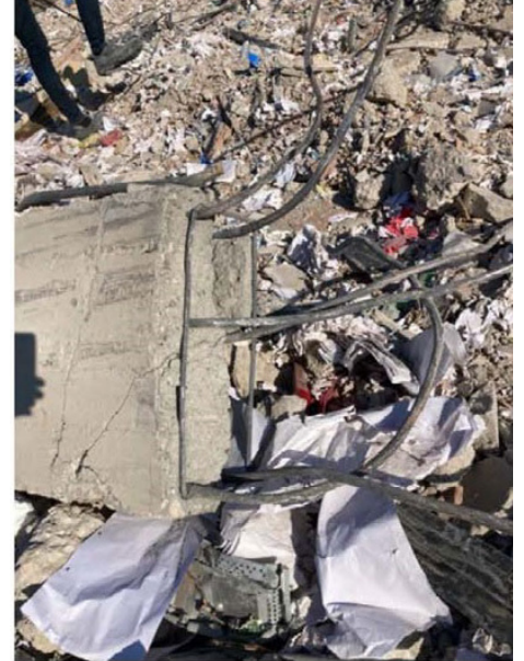
Enkaz alanında bir kolon parçası
